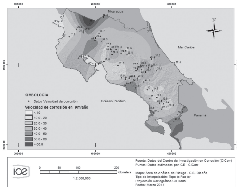
Fig. 8. Corrosión Atmosférica para acero de baja aleación según Modelado lineal con un año de mediciones del CICorr, en base a Cl , SO_2 y TDH ( \mu m \cdot a\tilde{no}^{-1} ).
