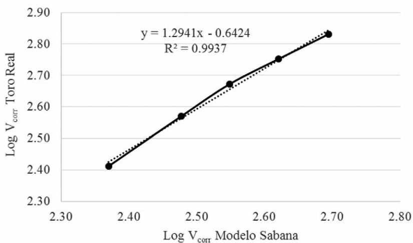
Figura 2. Relación entre \text{Log } V_{corr} ( \text{g x m}^{-2} ) obtenida con el modelo de Sabana, aplicando en ella los datos de Toro y su relación con los valores reales de \text{Log } V_{corr} ( \text{g x m}^{-2} ) obtenidos en Toro.
