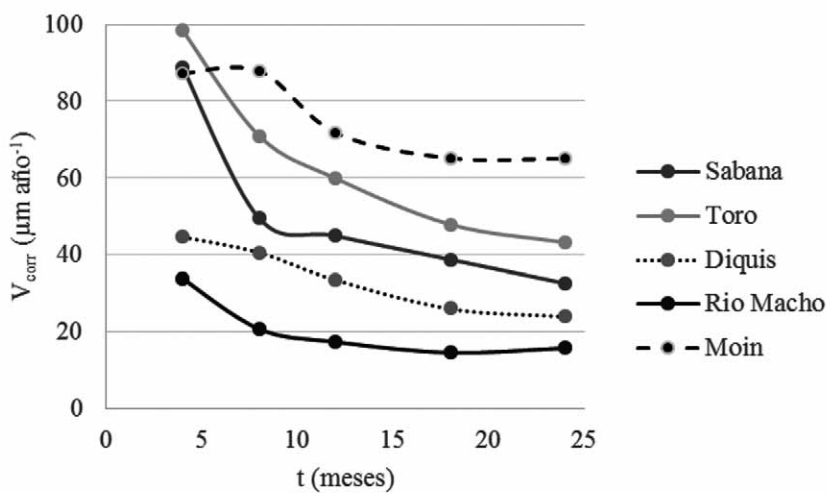
Figura 3. Evolución de V_{corr} ( \mu\text{m año}^{-1} ) con el tiempo para los 5 sitios analizados durante dos años.
