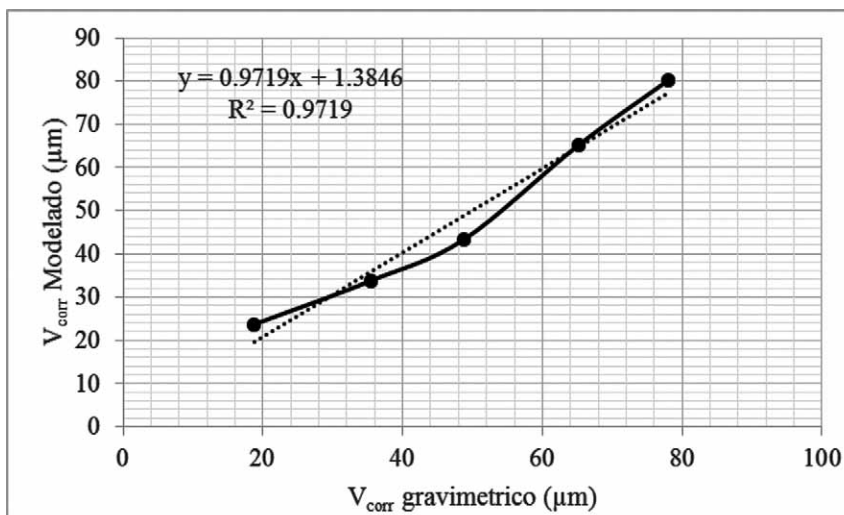
Figura 1. Relación entre la V_{corr} Modelado ( \mu\text{m} ) en el primer año calculada por la Ecuación 8, respecto a los valores de V_{corr} gravimétrico ( \mu\text{m} ) utilizados para el modelado.
